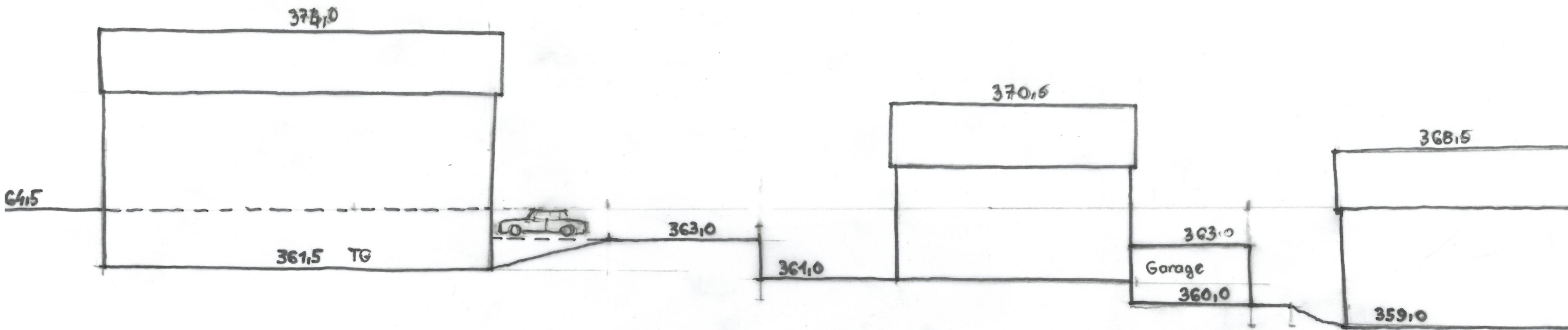
Schnitt V1
